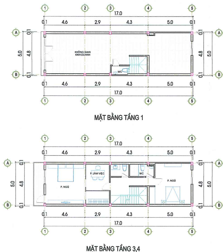
MẶT BẰNG NHÀ LIỀN KẾ ĐIỂN HÌNH (5X17M)
